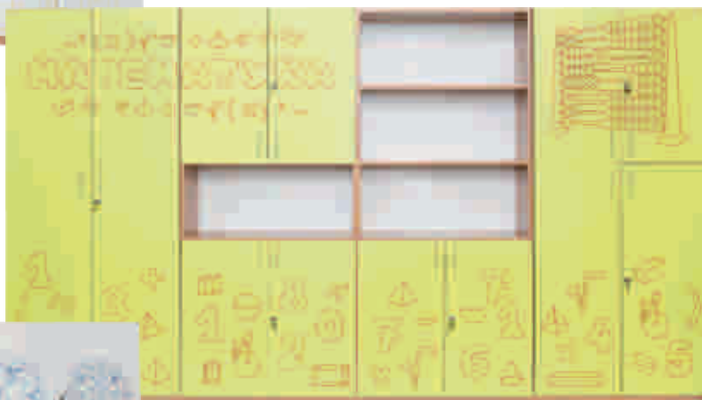
MATEMATYKA
