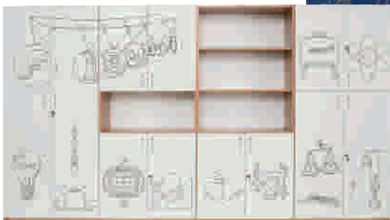
FIZYKA
