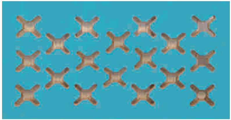
GWIAZDY
